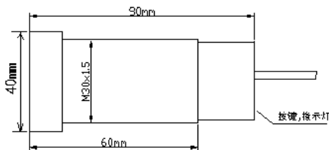
传感器后端
